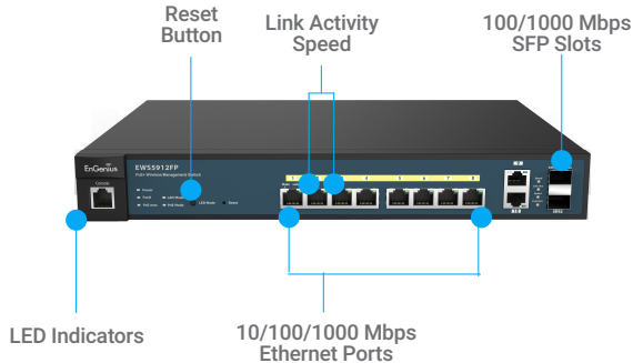
EWS5912FP
